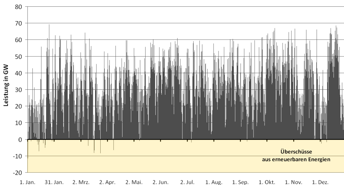
Residuallast des Übergangsszenarios 2.1.a im Jahr 2020
